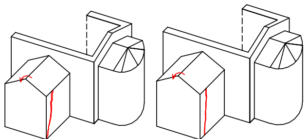
10. RIBALTAMENTO DELLE PARETI DI ESTREMITÀ
