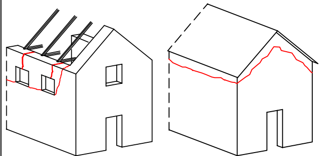
14. MARTELLAMENTO DELLA COPERTURA
