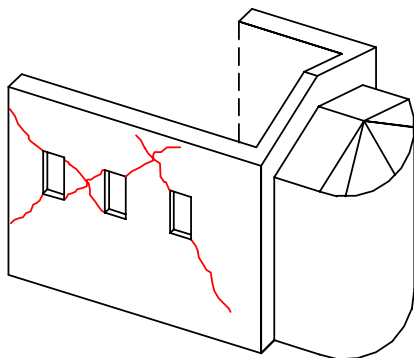
15. INTERAZIONI IN PROSSIMITA' DI IRREGOLARITA' PLANO-ALTIMETRICHE
