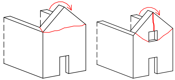
4. RISPOSTA TRASVERSALE DI AULA O TRANSETTO
