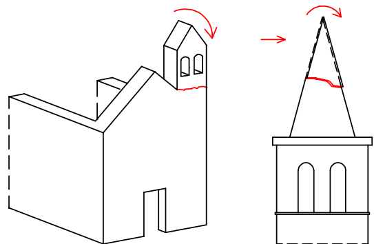
18. AGGETTI (VELA, GUGLIE, PINNACOLI, STATUE)
