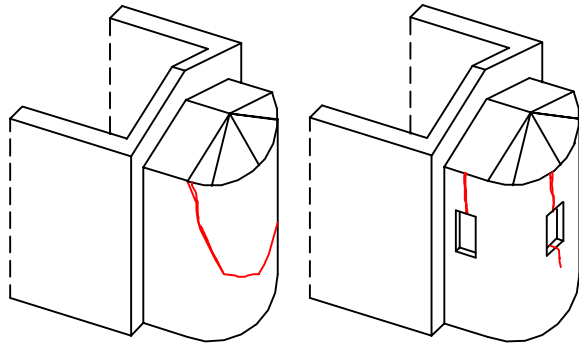
13. ROTTURA A TAGLIO DELLE PARETI
